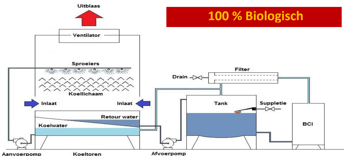
Voorbeeld koeltoren
